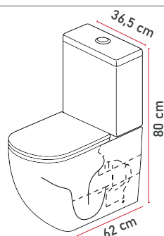
Esquema dimensiones
