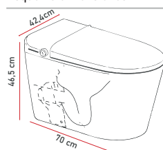
Esquema dimensiones
