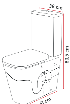
Esquema dimensiones
